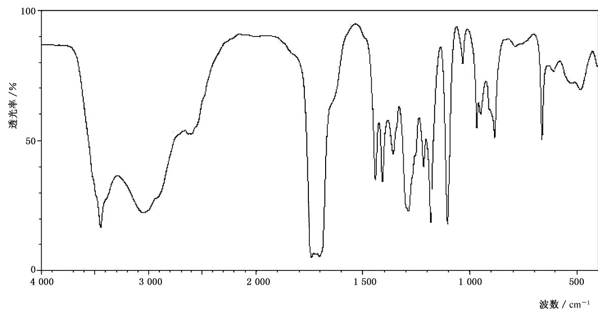
图 B.1 DL-苹果酸红外标准谱图
